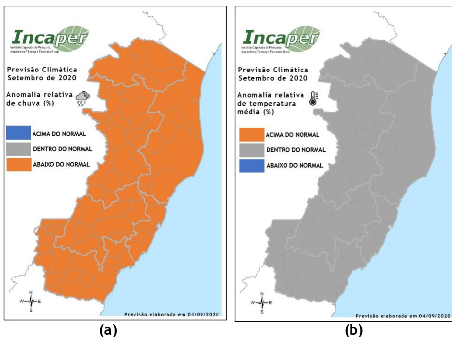
Figura 3. Prognóstico para setembro/2020: (a) precipitação e (b) temperatura média.
